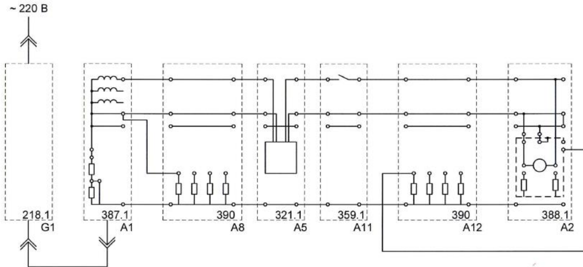
Рисунок 26 – Схема для подтверждения нецелесообразности применения УЗО в электроустановках с системой заземления TN-C.
