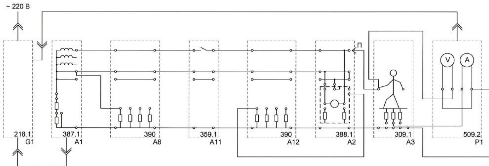
Рисунок 27 – Схема для подтверждения отсутствия защиты при прямом прикосновении человека к частям, находящимся под напряжением в электроустановках с системой заземления TN-C.
