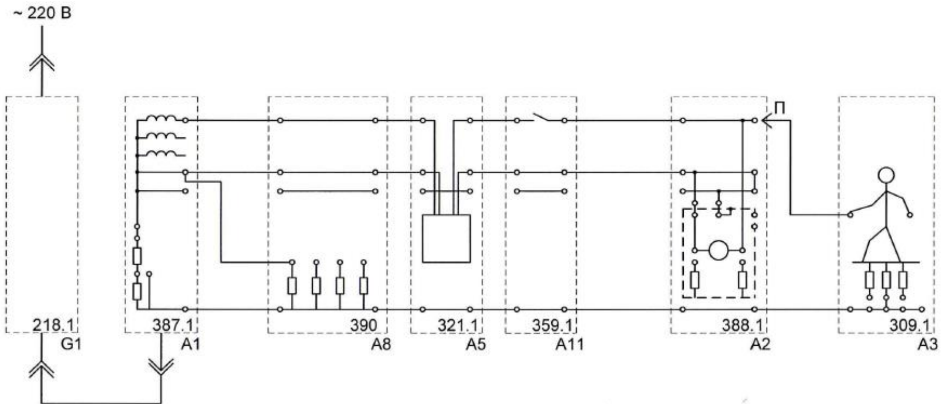
Рисунок 30 – Схема для выявления действия защиты при прямом прикосновении человека к частям, находящимся под напряжением в электроустановках с системой заземления TN-C.
