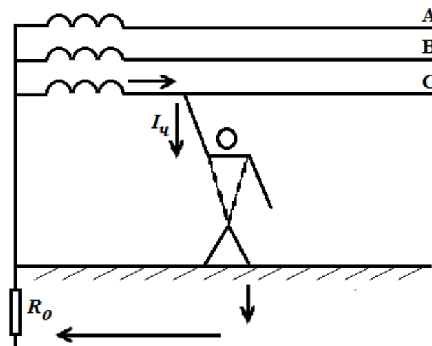
Рисунок 3 – Схема однофазного включения в сеть с заземленной нейтралью.
