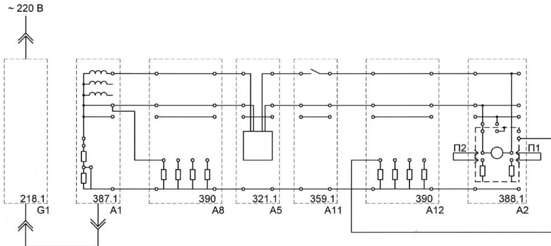
Рисунок 42 – Схема для выявления действия защиты при повреждении рабочей изоляции электроприёмника класса I в электроустановках до 1000 В с системой заземления ТТ (уменьшение сопротивления изоляции фазы до 15 кОм или – нулевого провода до 10 Ом)
