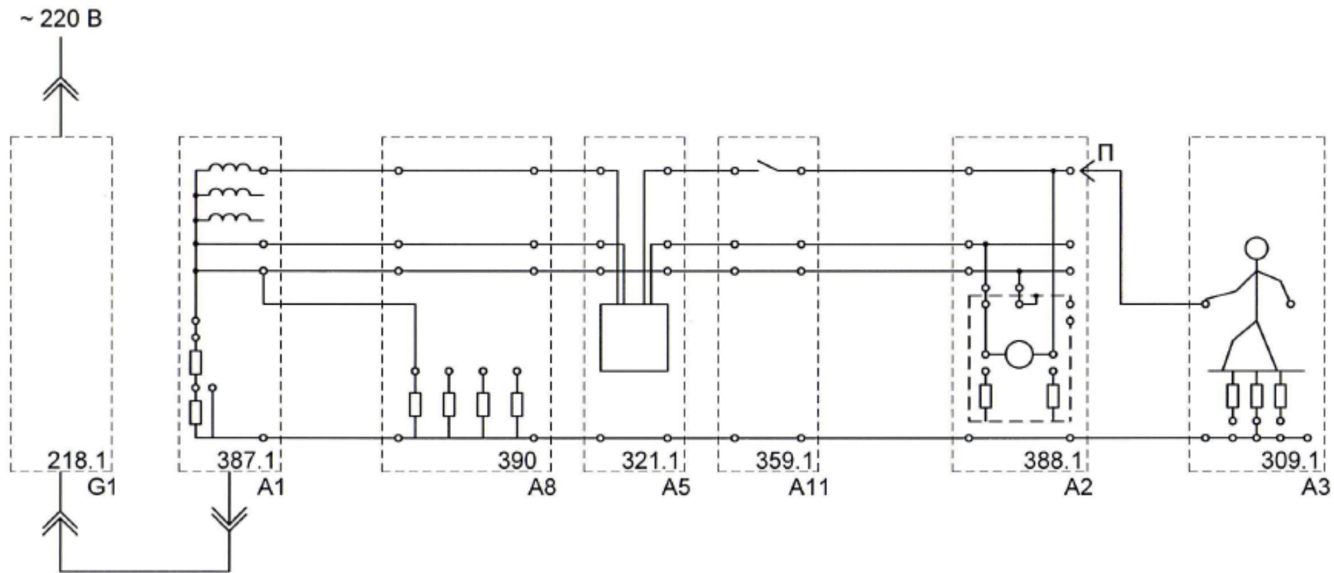
Рисунок 33 – Схема для выявления действия защиты при прямом прикосновении человека к частям, находящимся под напряжением в электроустановках до 1 кВ с системой заземления TN-S
