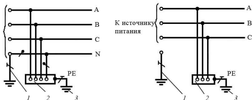
Рисунок 12– Система ТТ переменного тока при однофазном и трёхфазном электроприемниках (1 — заземлитель нейтрали источника переменного тока; 2 — открытые проводящие части; 3 — заземлитель открытых проводящих частей электроустановки;)
