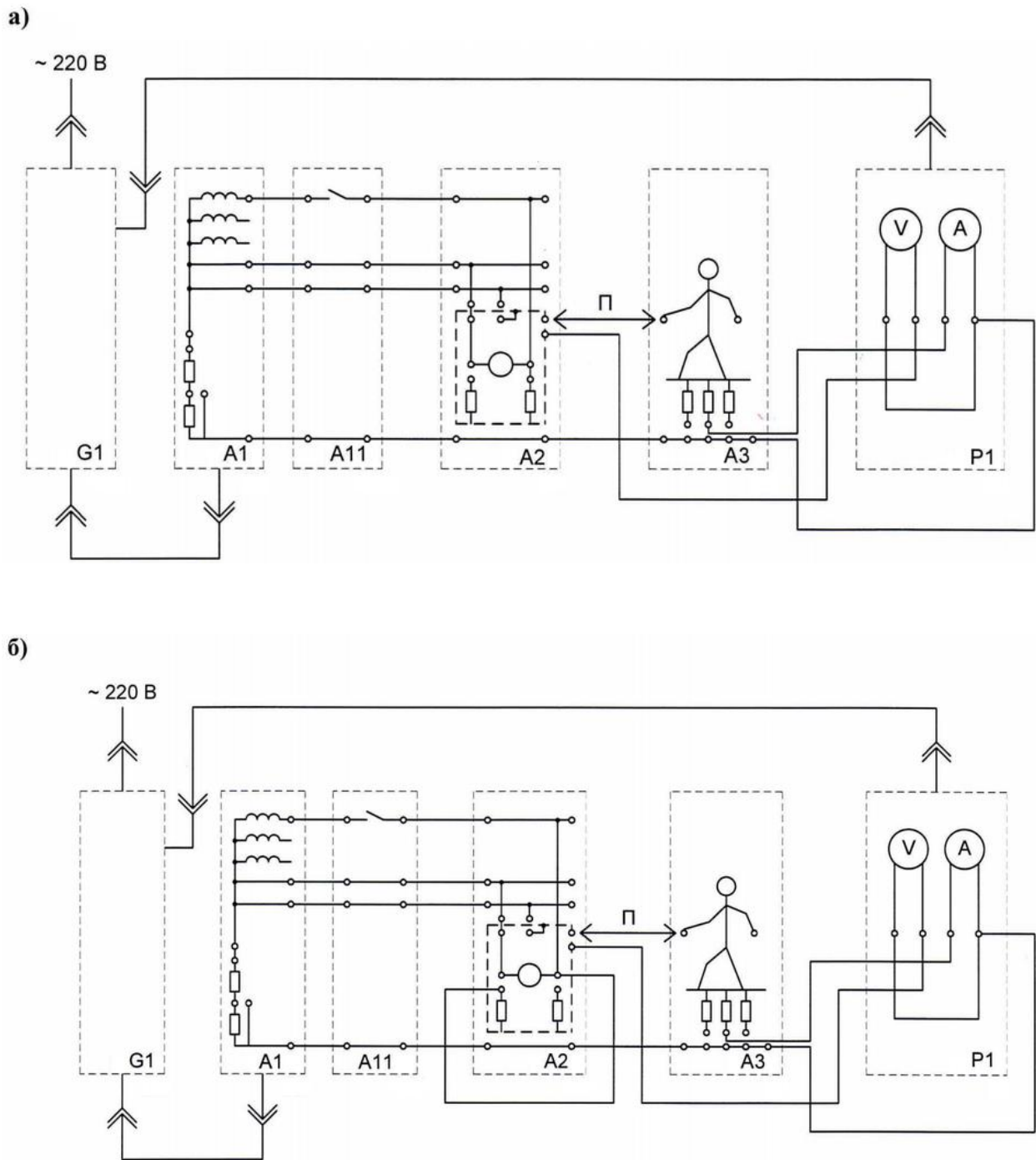
Рисунок 21 – Схема для определения силы тока, проходящего через тело человека при косвенном прикосновении к частям электрооборудования, находящимся под напряжением:
