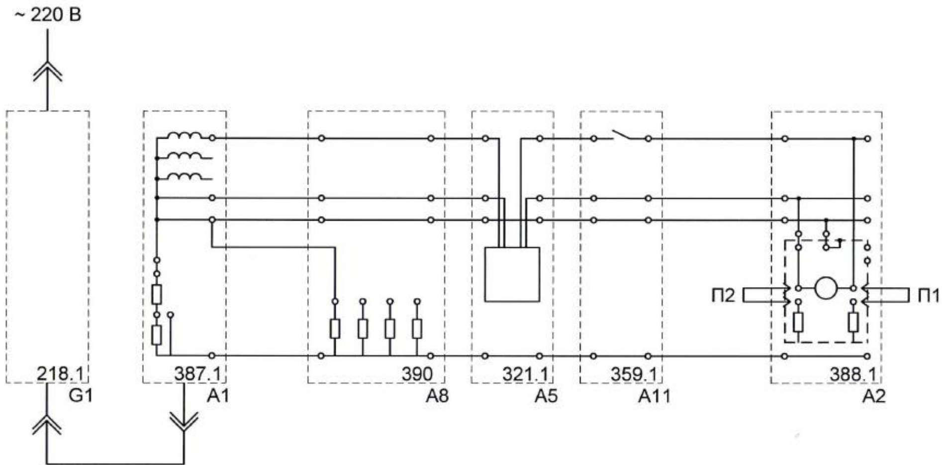
Рисунок 35 – Схема для выявления действия защиты при повреждении рабочей изоляции электроприёмника класса I в электроустановках до 1000 В с системой заземления TN-S (уменьшение сопротивления изоляции фазы до 15 кОм или – нулевого провода до 10 Ом)
