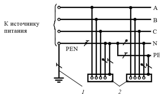
Рисунок 10 – Система TN-C-S переменного тока при однофазном и трёхфазном электроприемниках.
