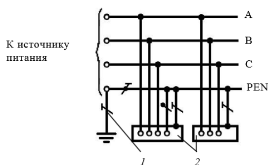
Рисунок 8 – Система TN-C переменного тока при однофазном и трёхфазном электроприемниках (1 — заземлитель нейтрали (средней точки) источника питания; 2 — открытые проводящие части).
