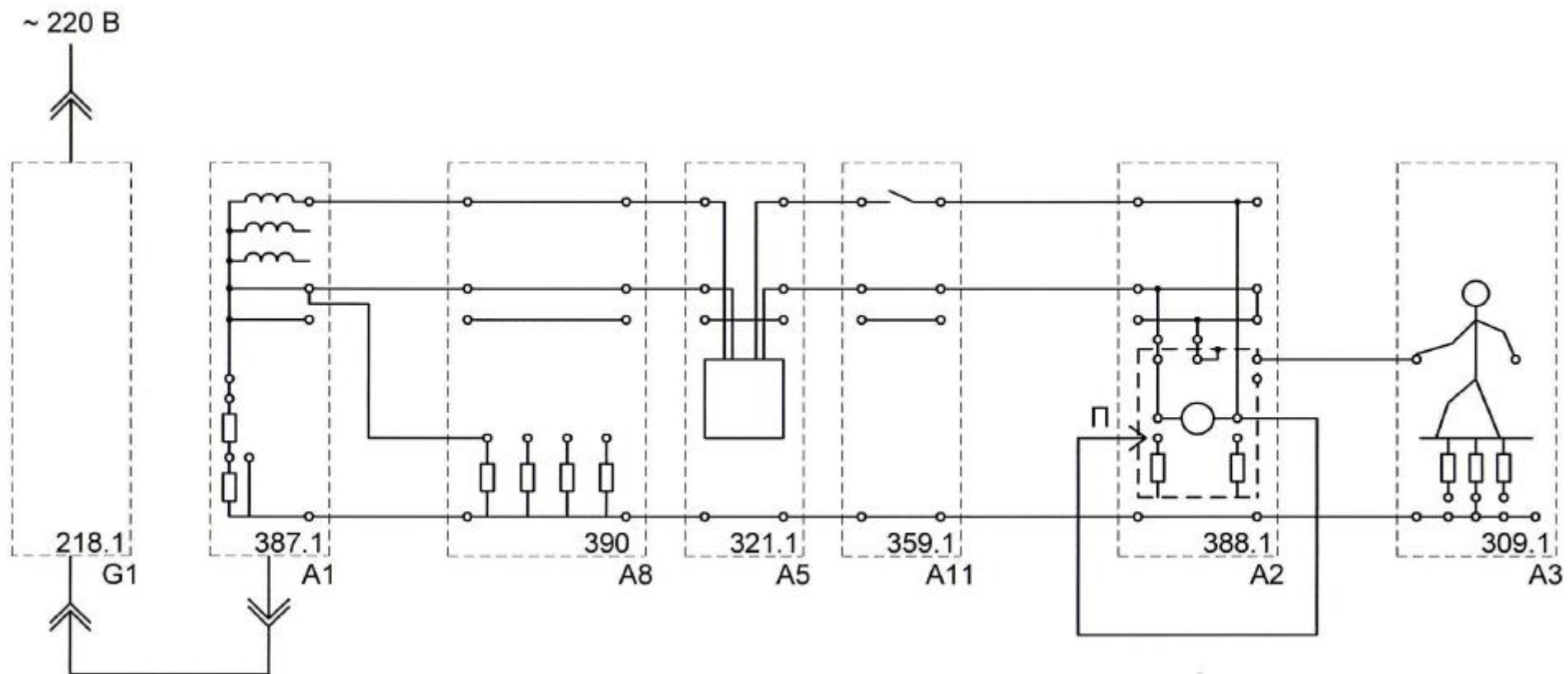
Рисунок 32 – Схема моделирования работы защиты при повреждении рабочей изоляции электроприёмника класса I в электроустановках с системой заземления TN-C (уменьшение сопротивления изоляции фазы до 15 кОм или – нулевого провода до 10 Ом)
