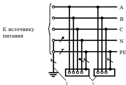
Рисунок 9 – Система TN-S переменного тока при однофазном и трёхфазном электроприемниках.
