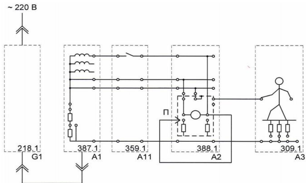
Рисунок 22 – Схема для выявления защитного действия устройства автоматического отключения питания при сверхтоках.
