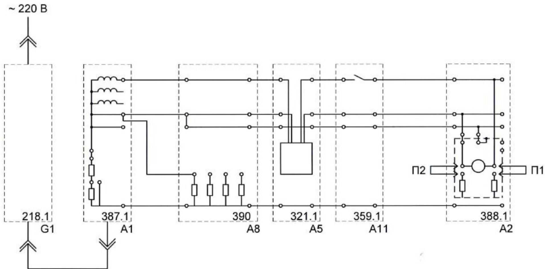
Рисунок 36 – Схема для выявления действия защиты при повреждении рабочей изоляции электроприёмника класса I в электроустановках до 1000 В с системой заземления TN-C-S (уменьшение сопротивления изоляции фазы до 15 кОм или – нулевого провода до 10 Ом)
