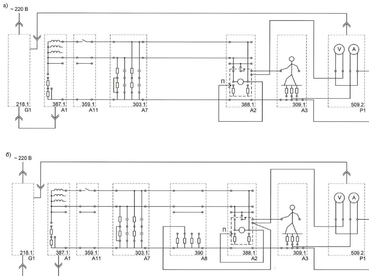
Рисунок 23 – Схема действия защитного заземления:
