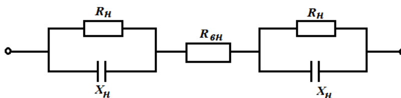
Рисунок 4 – Эквивалентная подробная схема замещения сопротивления тела человека.
