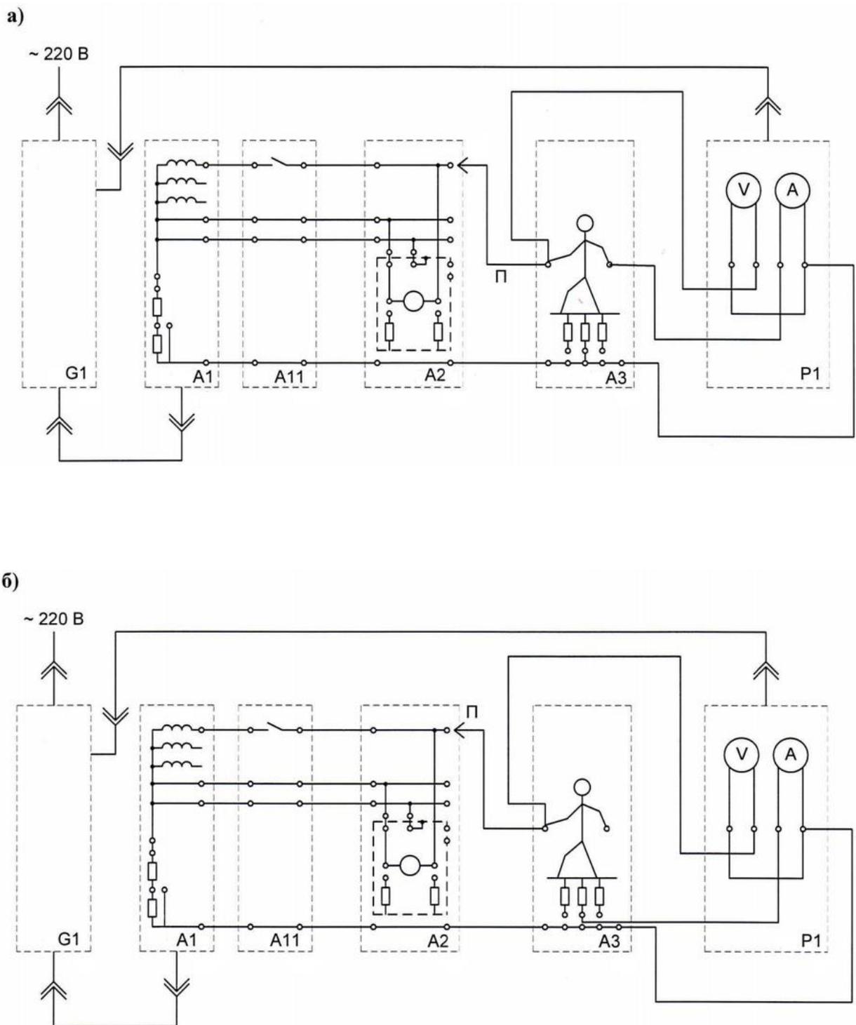
Рисунок 20 – Схема для определения силы тока, проходящего через тело человека при прямом прикосновении к частям электрооборудования, находящимся под напряжением:
