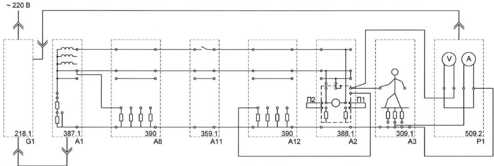
Рисунок 28– Схема моделирования работы защиты при повреждении рабочей изоляции электроприёмника класса I в электроустановках с системой заземления TN-C (уменьшение сопротивления изоляции фазы до 15 кОм или – нулевого провода до 10 Ом).
