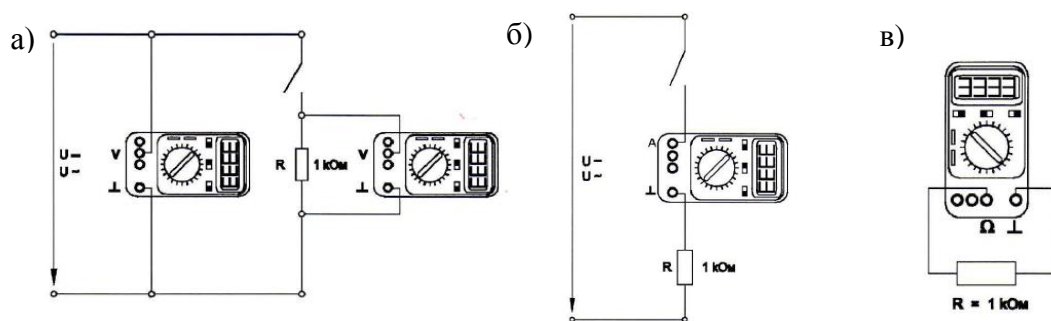
Рисунок 19 – Схемы включения мультиметра: а) как вольтметра; б) как амперметра; в) как омметра.
