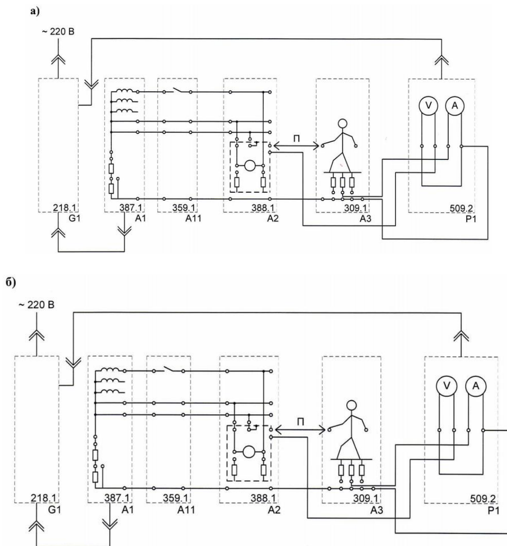
Рисунок 24 – Схема выявления защитного действия зануления:
