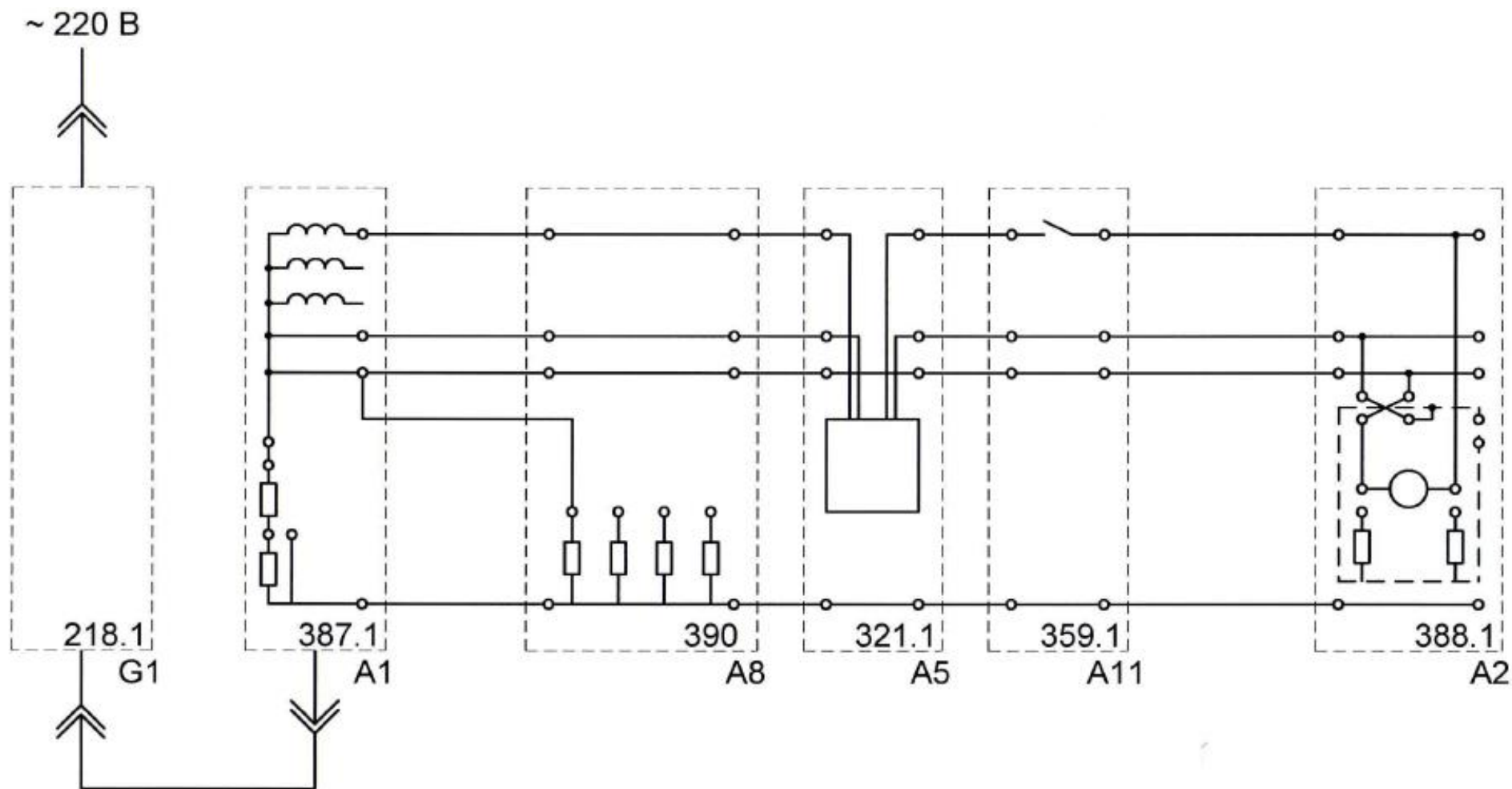
Рисунок 39 – Схема для выявления действия защиты при ошибочном присоединении нулевых рабочего и защитного проводников в электроустановках до 1000 В с системой заземления TN-S
