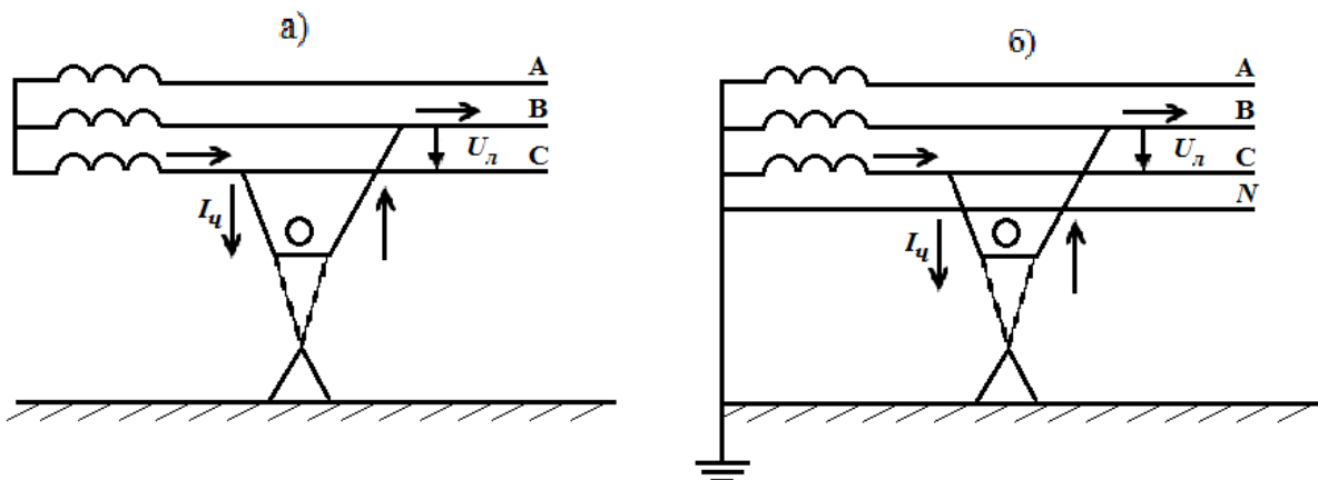
Рисунок 1 - Схема двухфазного включения человека в электрическую сеть: а – сеть с изолированной нейтралью; б – сеть с глухозаземленной нейтралью.
