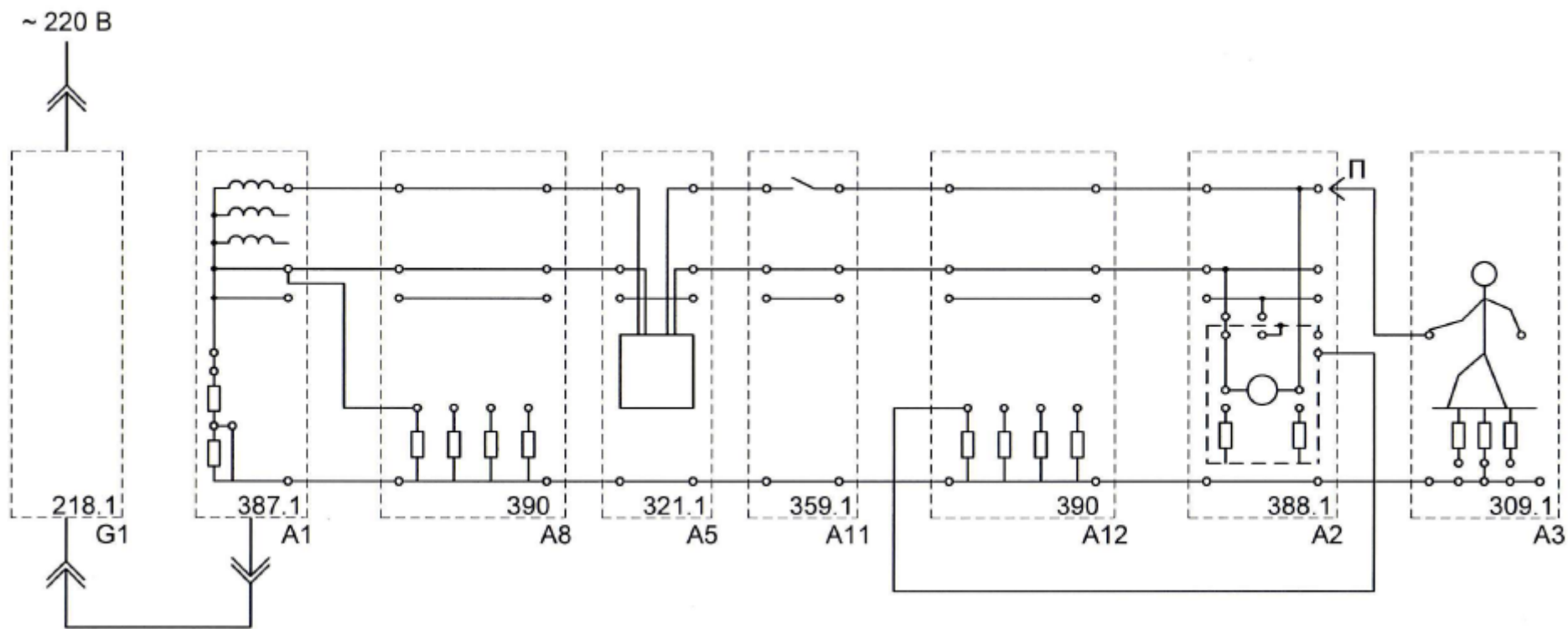
Рисунок 41 – Схема для выявления действия защиты при прямом прикосновении человека к частям, находящимся под напряжением в электроустановках с системой заземления ТТ.
