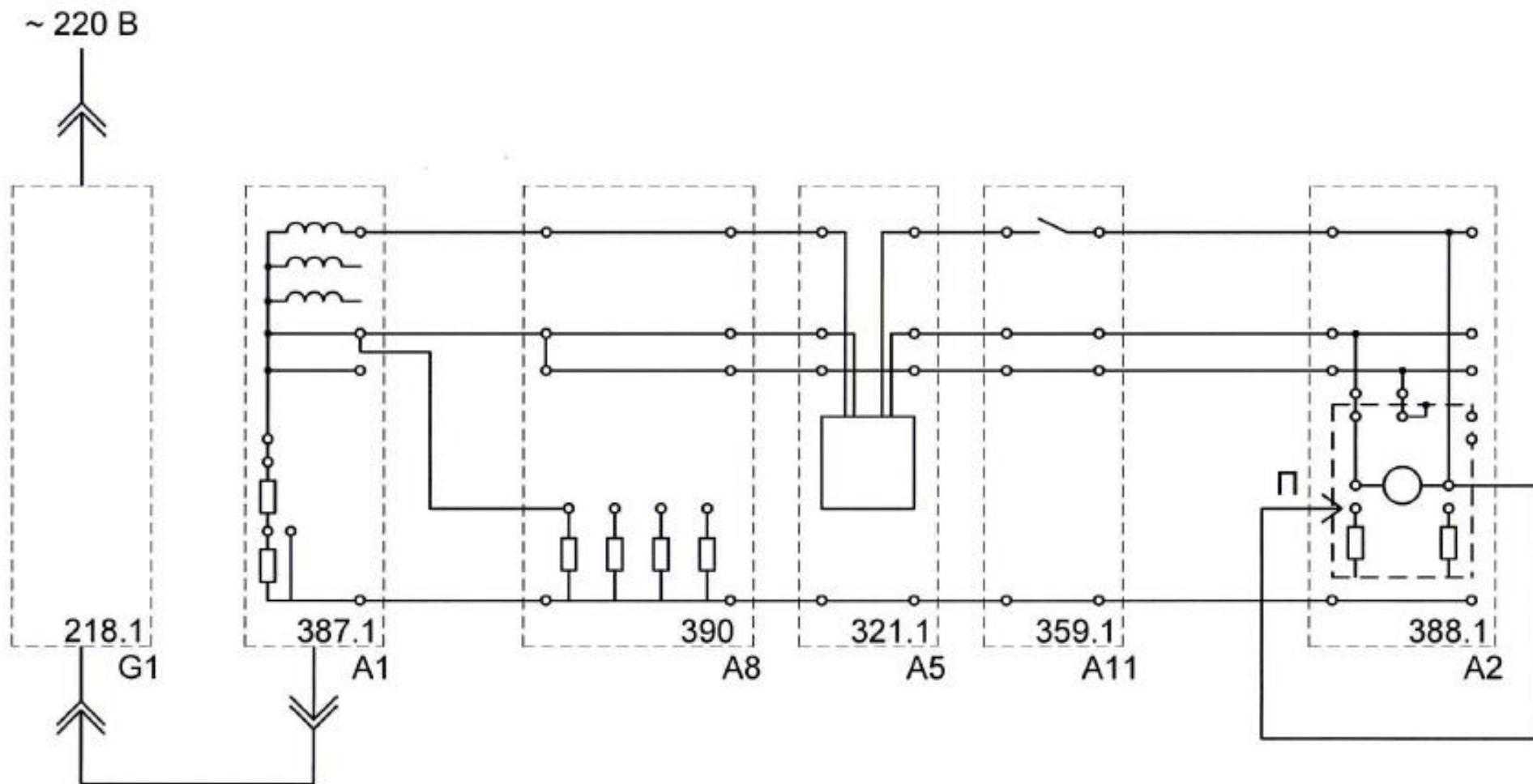
Рисунок 38 – Схема для выявления действия защиты при повреждении рабочей изоляции электроприёмника класса I в электроустановках до 1000 В с системой заземления TN-C-S (снижение сопротивления изоляции фазы до 10 кОм)
