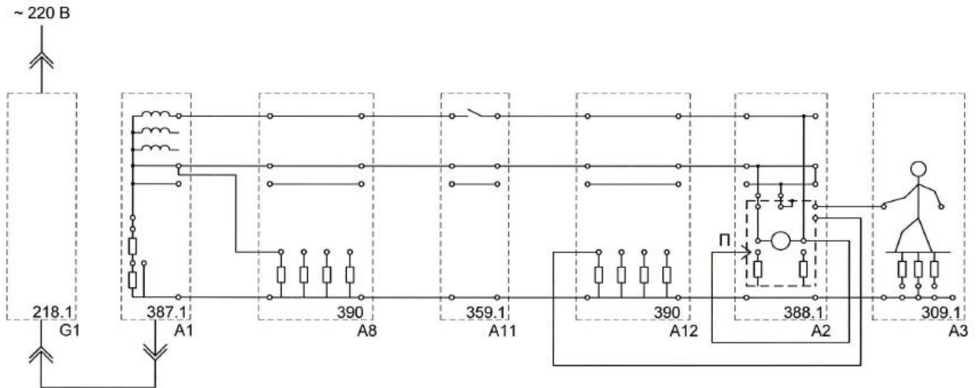
Рисунок 29 – Схема моделирования работы защиты при повреждении рабочей изоляции электроприёмника класса I в электроустановках с системой заземления TN-C (уменьшение сопротивления изоляции фазы до 10).
