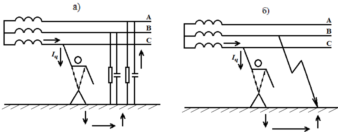
Рисунок 2 - Схема однофазного включения в сеть с изолированной нейтралью: а – при хорошей изоляции; б – при аварийном режиме.
