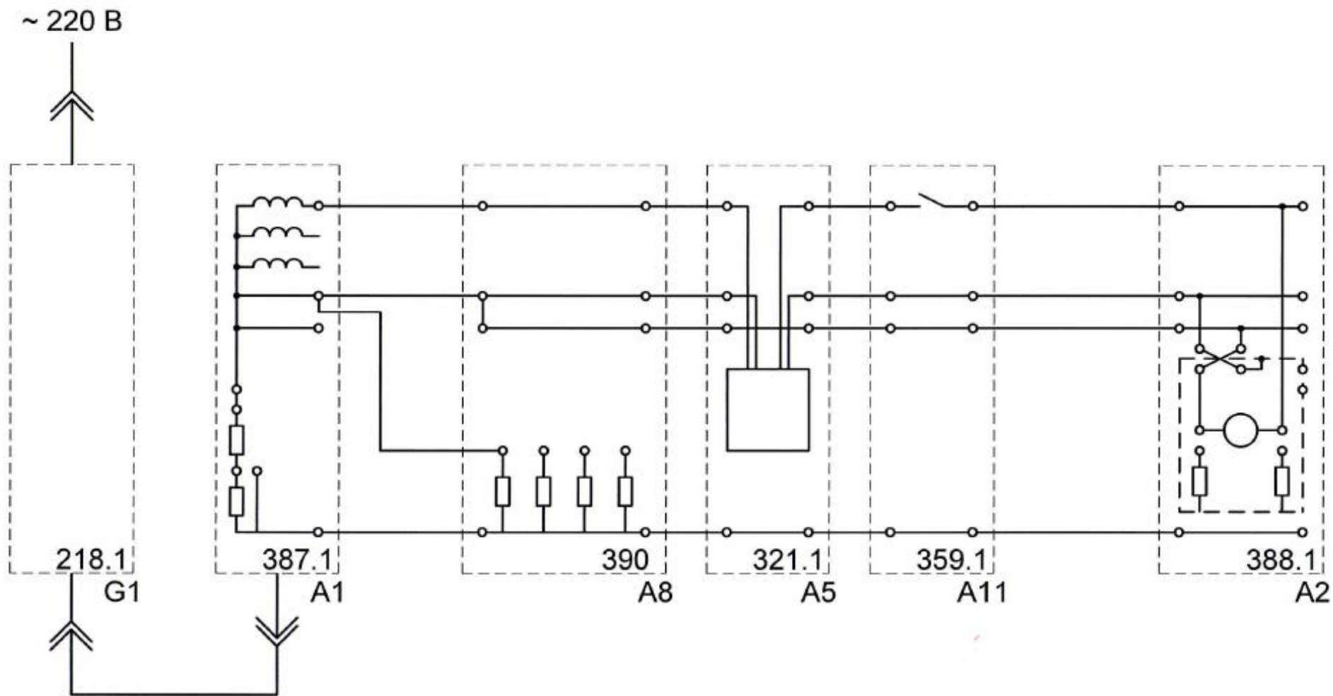
Рисунок 40 – Схема для выявления действия защиты при ошибочном присоединении нулевых рабочего и защитного проводников в электроустановках до 1000 В с системой заземления TN-C-S
