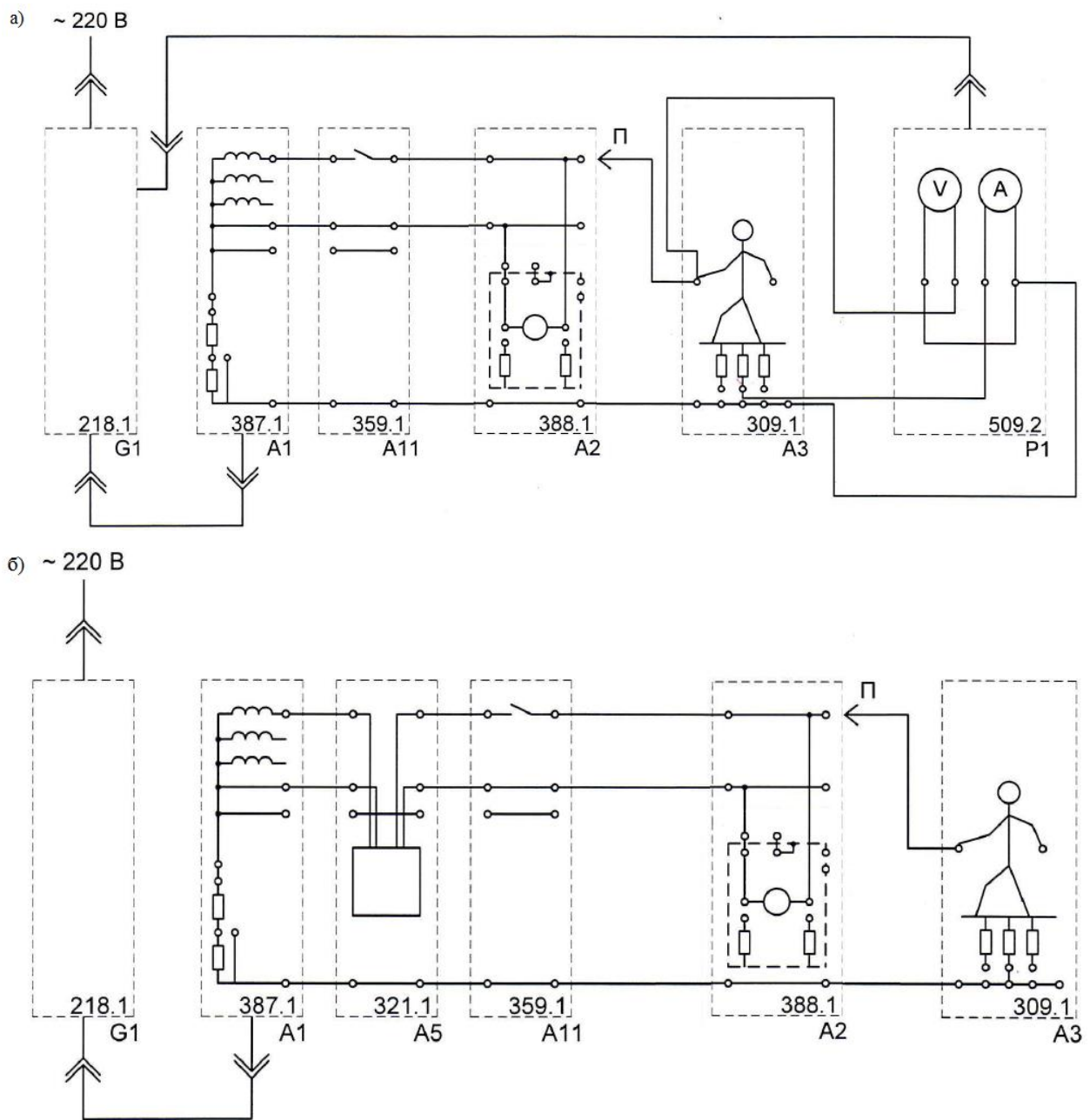
Рисунок 25 – Схема для выявления действия устройства защитного отключения: а) без УЗО; б) с УЗО.
