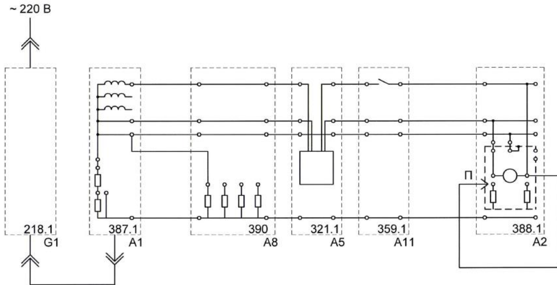
Рисунок 37 – Схема для выявления действия защиты при повреждении рабочей изоляции электроприёмника класса I в электроустановках до 1000 В с системой заземления TN- S (снижение сопротивления изоляции фазы до 10 кОм)
