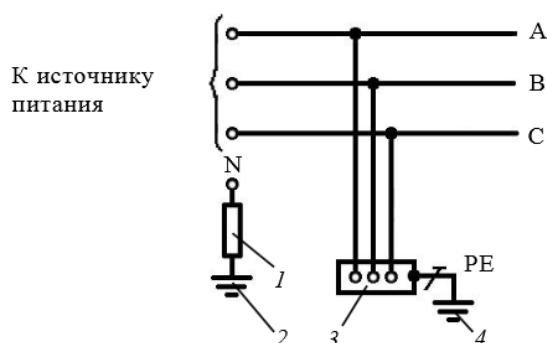
Рисунок 11 – Система IT переменного тока при однофазном и трёхфазном электроприемниках (1 — сопротивление заземления нейтрали источника питания; 2 — заземлитель; 3 — открытые проводящие части; 4 — заземляющее устройство электроустановки)
