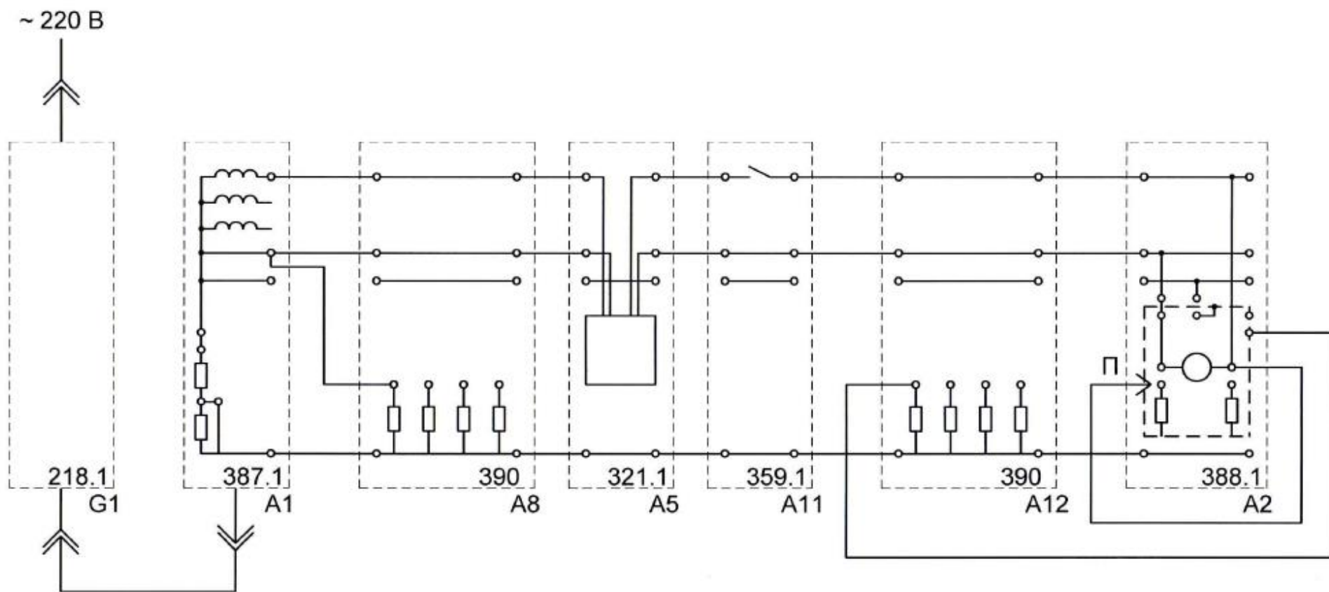
Рисунок 43 – Схема для выявления действия защиты при повреждении рабочей изоляции электроприёмника класса I в электроустановках до 1000 В с системой заземления ТТ (снижение сопротивления изоляции фазы до 10 кОм)
